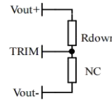
电压下调: 在Trim和输出正之间增加电阻Rdown
